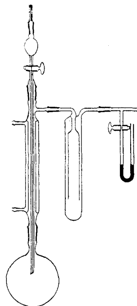
Fig. 1.—Apparatus.
